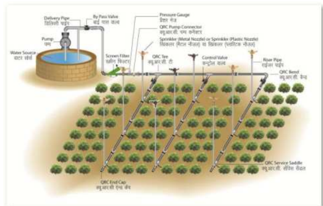
Layout of Sprinkler Irrigation System (सिंचन प्रणाली का रखांक)
